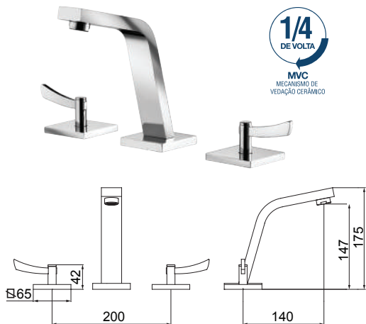
1877 C67 MISTURADOR PARA LAVATÓRIO DE MESA BICA ALTA
