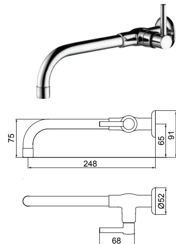
1161 C31 TORNEIRA PARA LAVATÓRIO DE PAREDE
