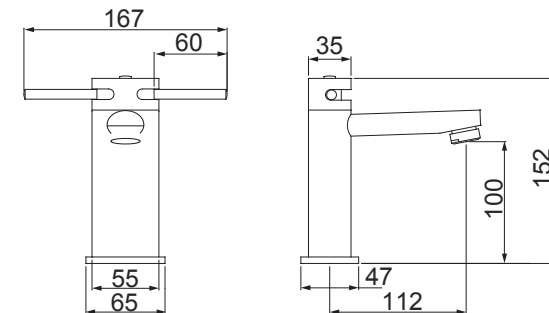
3875 C66 MISTURADOR MONOBLOCO PARA LAVATÓRIO DE MESA
