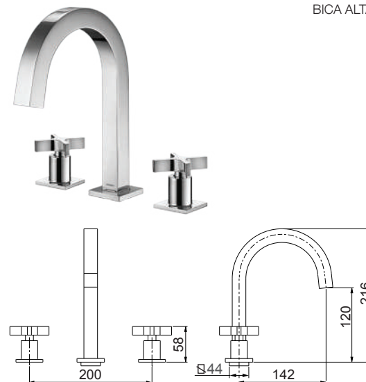
1876 C88 MISTURADOR PARA LAVATÓRIO DE MESA BICA ALTA
