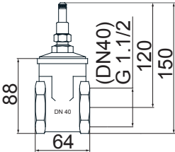
BASE DE REGISTRO DE GAVETA DN40 1 1/2
