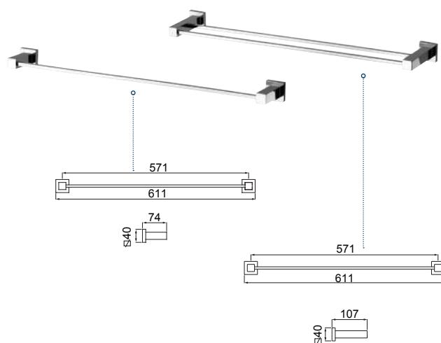
2042 C84 TOALHEIRO BARRA DUPLO
