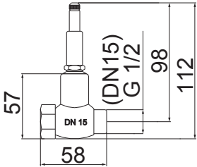
BASE DE REGISTRO DE PRESSÃO DN15 1/2
