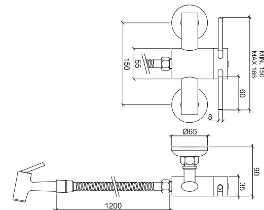
1982 C66 MISTURADOR DUCHA HIGIÊNICA FLEXÍVEL DE 1,20M GATILHO EM METAL
