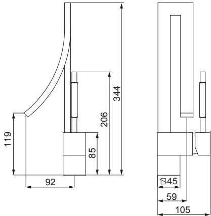
2875 C77 MISTURADOR MONOCOMANDO PARA LAVATÓRIO DE MESA
