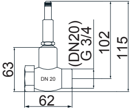
BASE DE REGISTRO DE PRESSÃO DN20 3/4
