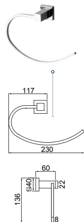
2050 C84 TOALHEIRO ARGOLA
