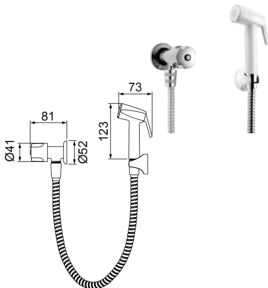
1984 C28 DUCHA HIGIÊNICA | FLEXÍVEL DE 1,20M
