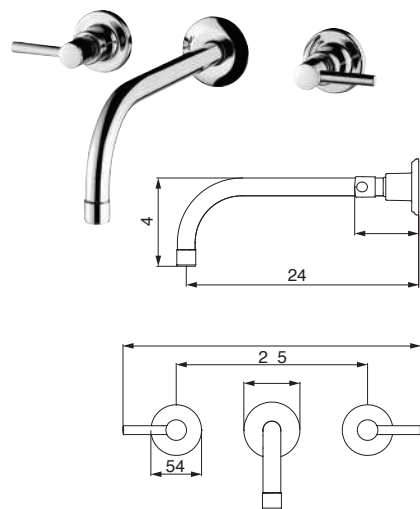
1878 C31 MISTURADOR PARA LAVATÓRIO DE PAREDE
