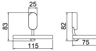
2040 C32 TOALHEIRO BARRA
