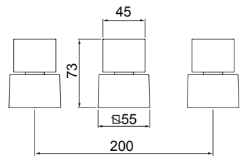
1895 C84 MISTURADOR PARA BIDÊ
