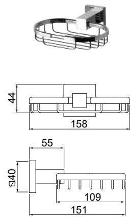
2008 C84 SABONETEIRA CESTO DE METAL
