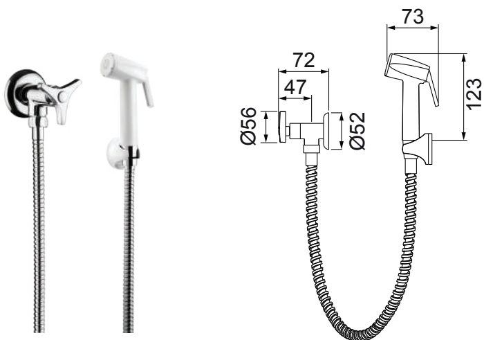
1984 C30 DUCHA HIGIÊNICA | FLEXÍVEL DE 1,20M
