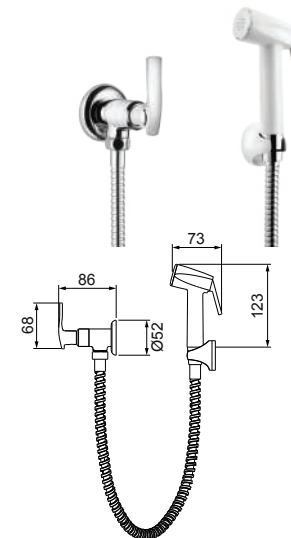
1984 C29 DUCHA HIGIÊNICA | FLEXÍVEL DE 1,20M
