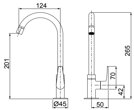
1877 C32 MISTURADOR PARA LAVATÓRIO DE MESA BICA ALTA
