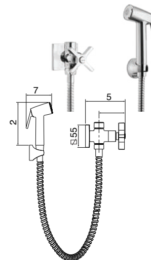
1984 C88 DUCHA HIGIÊNICA FLEXÍVEL DE 1,20M
