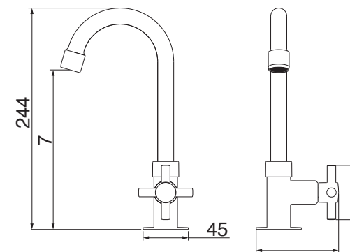
1878 C34 MISTURADOR PARA LAVATÓRIO DE PAREDE
