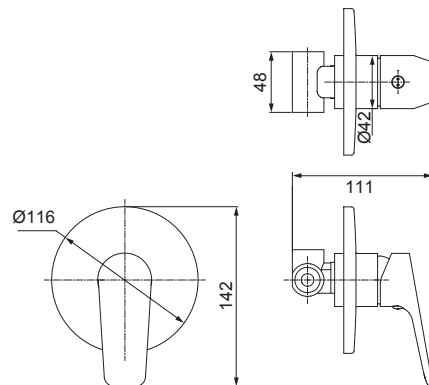
2993 C72 MONOCOMANDO PARA CHUVEIRO COM BASE 1/2"
