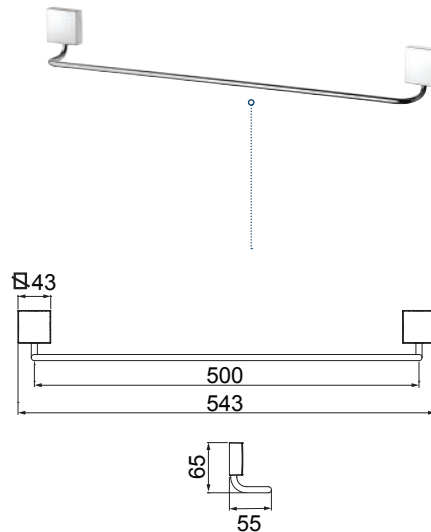
2040 C67 TOALHEIRO BARRA
