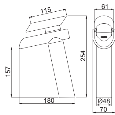
2877 C75 MISTURADOR MONOCOMANDO LAVATÓRIO PARA CUBA DE APOIO
