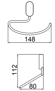
2000 C32 KIT DE ACESSÓRIOS PARA BANHEIRO: TOALHEIRO BARRA TOALHEIRO ARGOLA SABONETEIRA PAPELEIRA CABIDE
