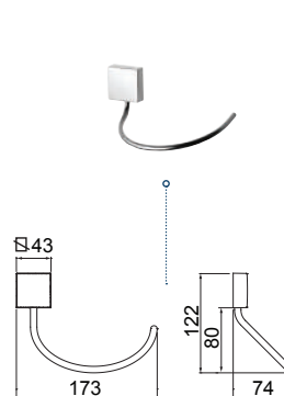
2050 C67 TOALHEIRO ARGOLA
