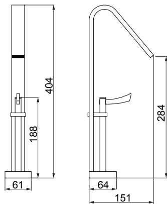
4877 C67 MISTURADOR MONOMIX LAVATÓRIO PARA CUBA DE APOIO
