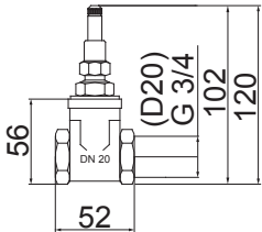
BASE DE REGISTRO DE GAVETA DN20 3/4
