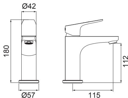
2875 C90 MISTURADOR MONOCOMANDO PARA LAVATÓRIO DE MESA
