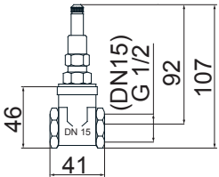
BASE DE REGISTRO DE GAVETA DN15 1/2
