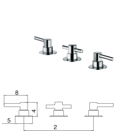
1895 C31 MISTURADOR PARA BIDÊ
