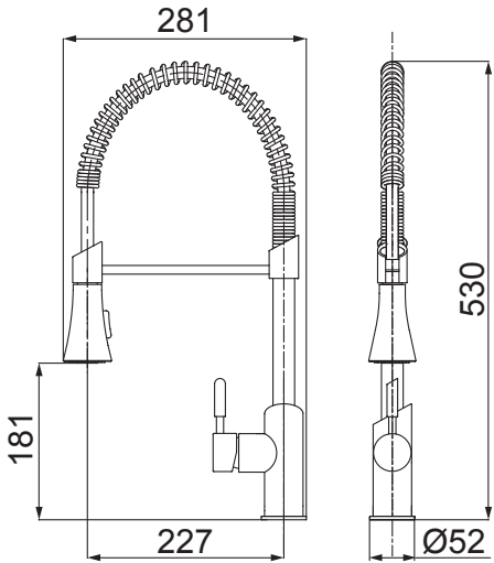
2266 C76 MISTURADOR MONOCOMANDO PARA COZINHA DE MESA COM DUCHA ESPECIAL
