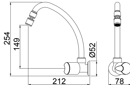
1167 C41 TORNEIRA PARA COZINHA DE MESA BICA MÓVEL
