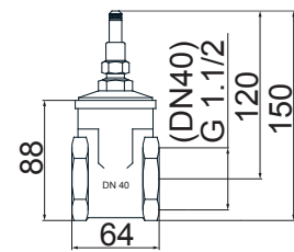
1500 C10 BASE DE REGISTRO DE GAVETA DN40 1 1/2"
