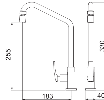
1167 C78 TORNEIRA PARA COZINHA DE MESA BICA MÓVEL
