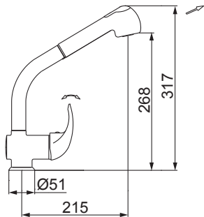
2267 C71 MISTURADOR MONOCOMANDO PARA COZINHA DE MESA BICA ALTA MÓVEL SPRAY
