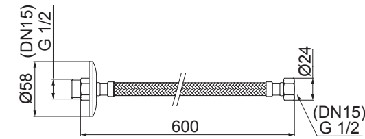
1794 C18 FLEXÍVEL TRANÇADO AÇO INOX ALTA PRESSÃO DN15(1/2") X 60CM INDICADO PARA ÁGUA QUENTE E FRIA DE LAVATÓRIOS, PIAS E BIDÊS. INDICADO PARA LIGAÇÕES DE ÁGUA QUENTE E FRIA DE AQUECEDORES DE ÁGUA A GÁS. OPÇÃO DE COR: CROMADO
