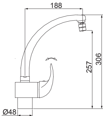
2257 C71 MISTURADOR MONOCOMANDO PARA COZINHA DE MESA BICA ALTA MÓVEL
