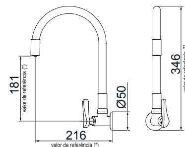
TORNEIRA MULTIUSO DE PAREDE BICA FLEXÍVEL
