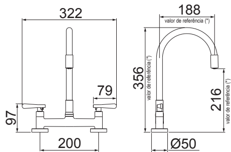
MISTURADOR PARA COZINHA DE MESA BICA FLEXÍVEL
