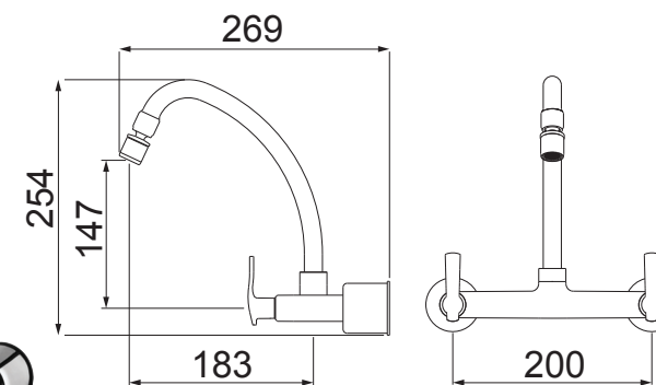
1258 C29 MISTURADOR PARA COZINHA DE PAREDE BICA MÓVEL
