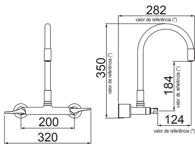
MISTURADOR PARA COZINHA DE PAREDE BICA FLEXÍVEL
