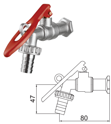
1127 C12 TORNEIRA DE ESFERA PARA CADEADO
