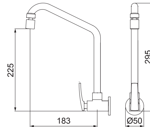
1168 C78 TORNEIRA PARA COZINHA DE PAREDE BICA MÓVEL
