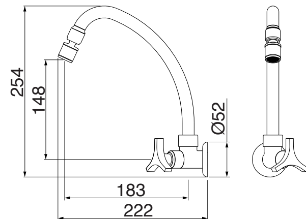
1168 C33 TORNEIRA PARA COZINHA DE PAREDE BICA MÓVEL
