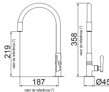
TORNEIRA MULTIUSO DE MESA BICA FLEXÍVEL
