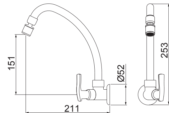
1258 C29 MISTURADOR PARA COZINHA DE PAREDE BICA MÓVEL
