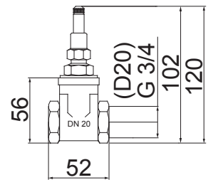
1500 C10 BASE DE REGISTRO DE GAVETA DN20 3/4"
