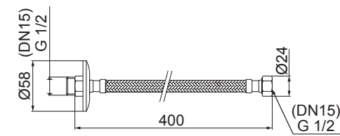
1792 C18 FLEXÍVEL TRANÇADO AÇO INOX ALTA PRESSÃO DN15(1/2") X 40CM INDICADO PARA ÁGUA QUENTE E FRIA DE LAVATÓRIOS, PIAS E BIDÊS. INDICADO PARA LIGAÇÕES DE ÁGUA QUENTE E FRIA DE AQUECEDORES DE ÁGUA A GÁS. OPÇÃO DE COR: CROMADO
