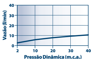
Curva de Vazão x Pressão da Ducha
