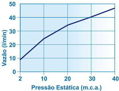
Curva de Vazão x Pressão da Ducha
